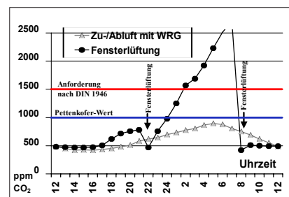
Vergleich Fensterlüftung und ventilatorgestützte Lüftung: Die CO 2 -Belastung übersteigt bei manueller Lüftung in einem Schlafzimmer nachts die Anforderungswerte deutlich.
